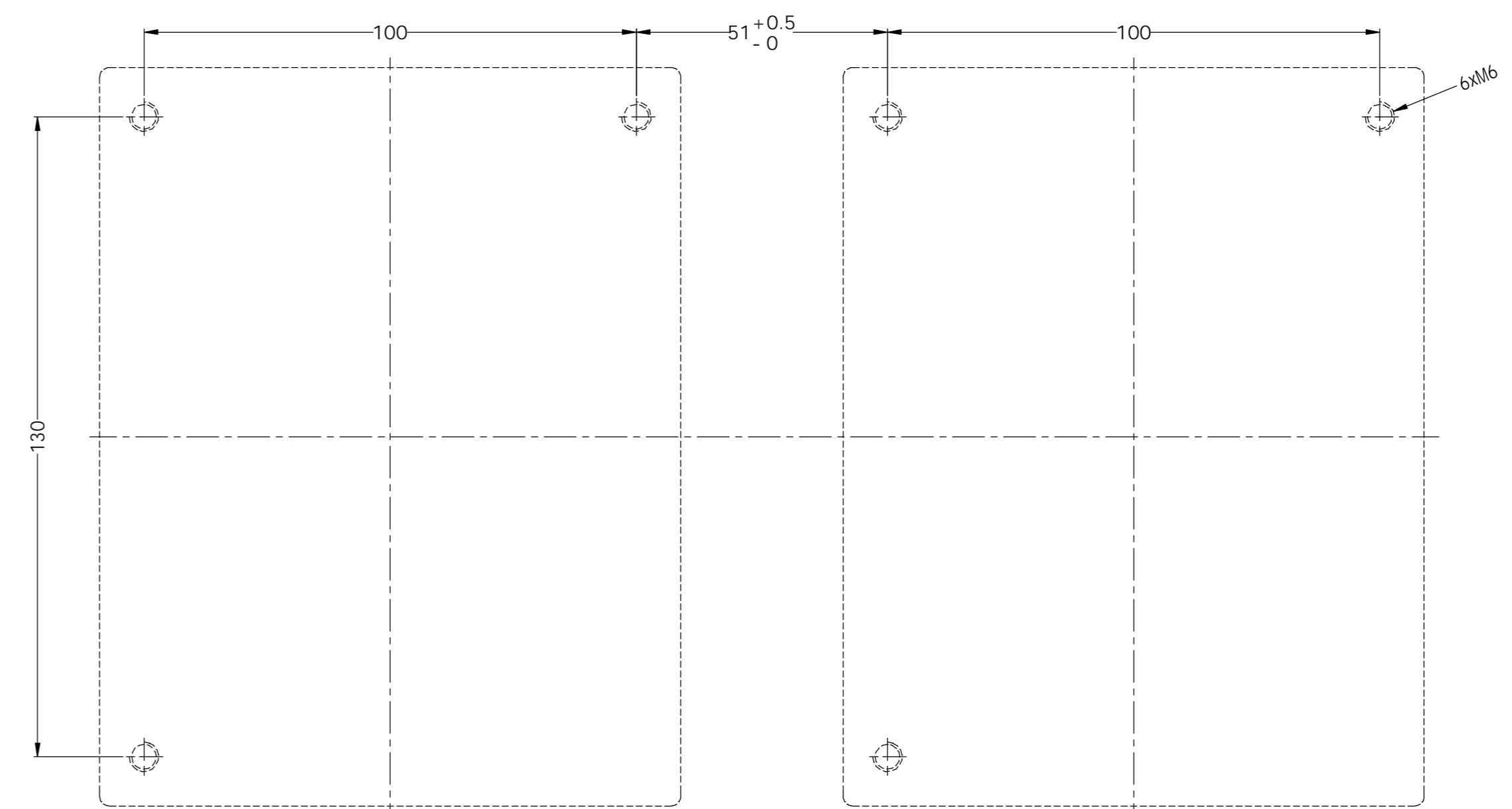
Dimensões para fixação dos contatores intertravados sem placa
