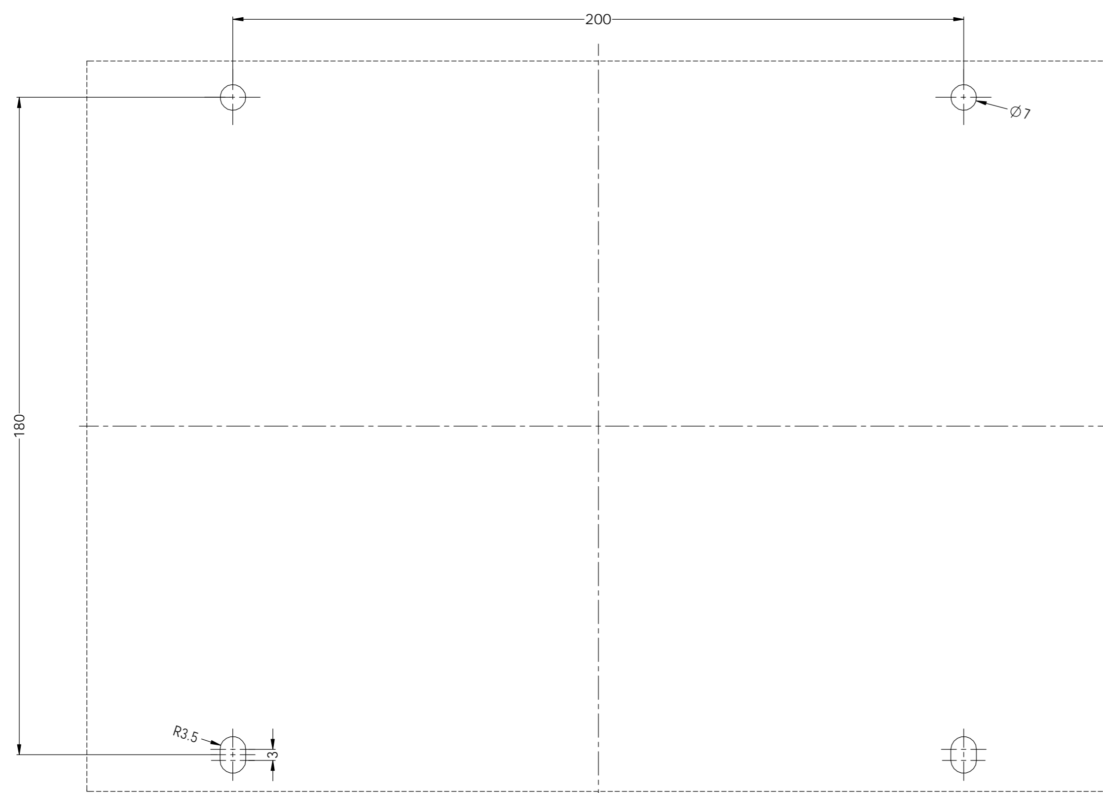
Dimensões para fixação dos contatores intertravados com placa
